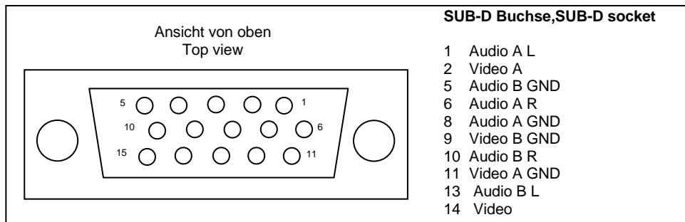
Bild 6 SUB-D Anschlussbelegung
